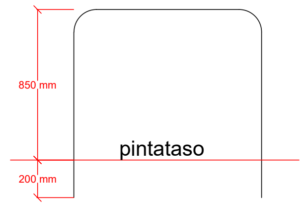
PERIAATEKUVA UPPOASENNUKSESTA (MITAT RIIPPUU VALMISTAJASTA)
